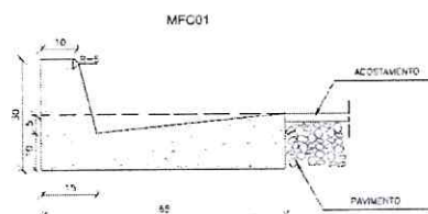
Figura 1: Modelo de Sarjeta segundo DNIT
