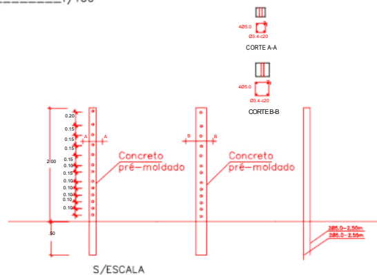
FACHADA CERCA ESCALA _____ 1/100
