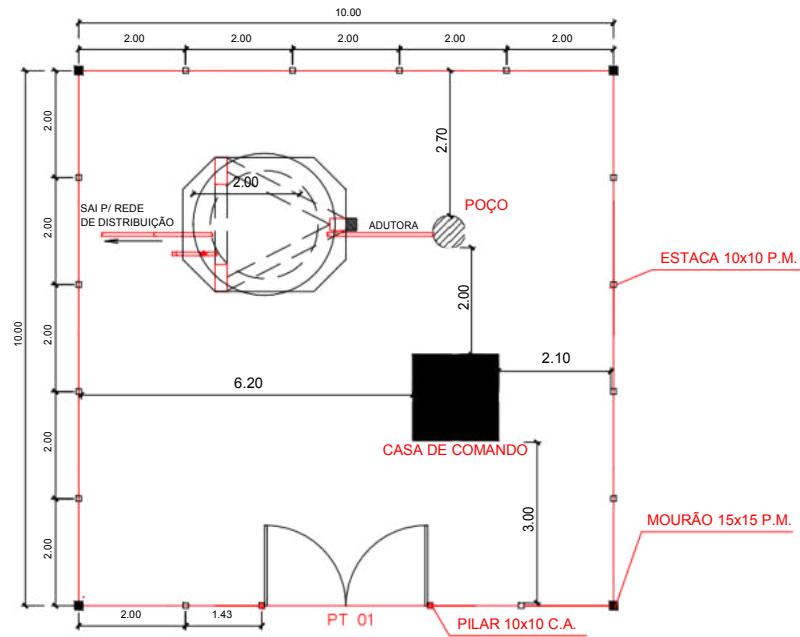
PLANTA DE SITUAÇÃO E LOCAÇÃO DO POÇO / RESERVATÓRIO E CASA DE COMANDO ESCALA _____ 1/100
